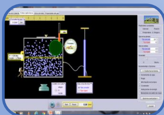
Procesos Termodinámicos
