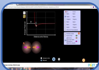
Interacción Atómica
