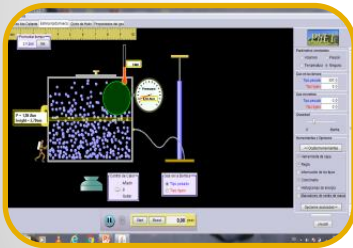
Procesos Termodinámicos
