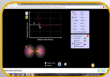
Interacción Atómica
